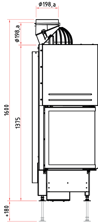
Seitenansicht M 1:20
